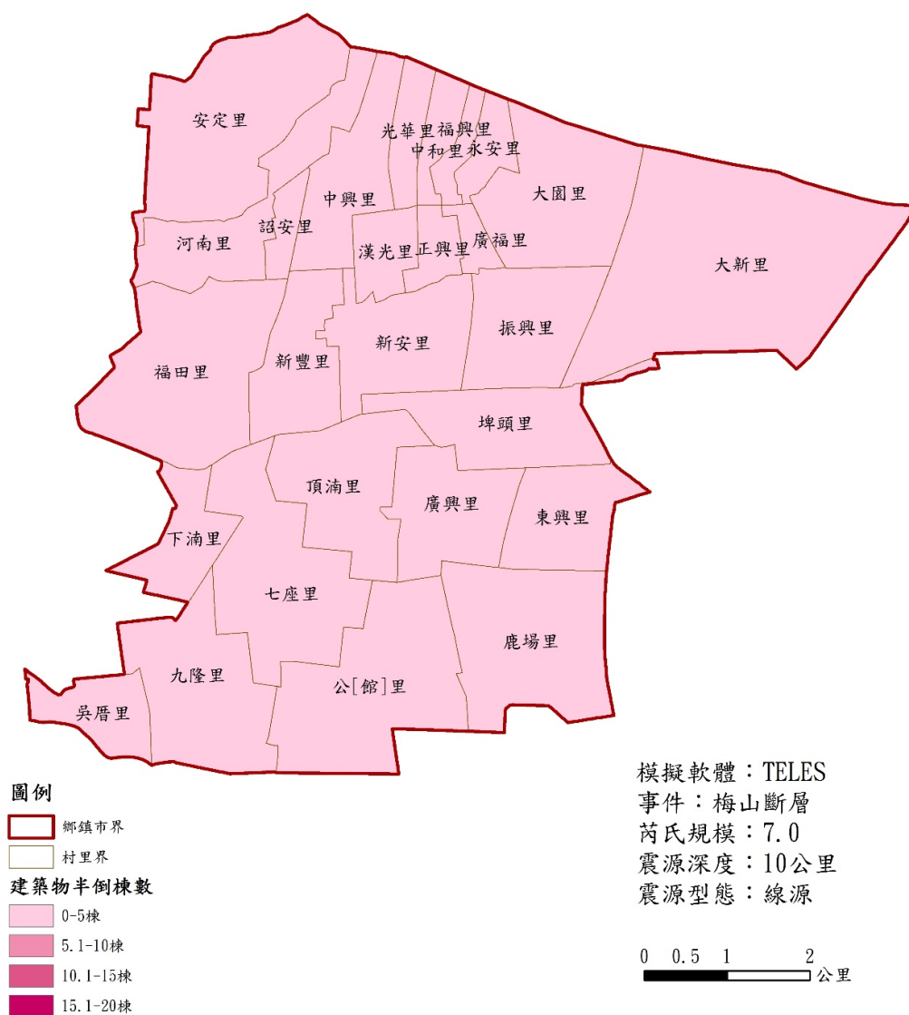
圖 1-4-5 西螺鎮地震災害潛勢圖(建築物倒塌棟數-半倒)
