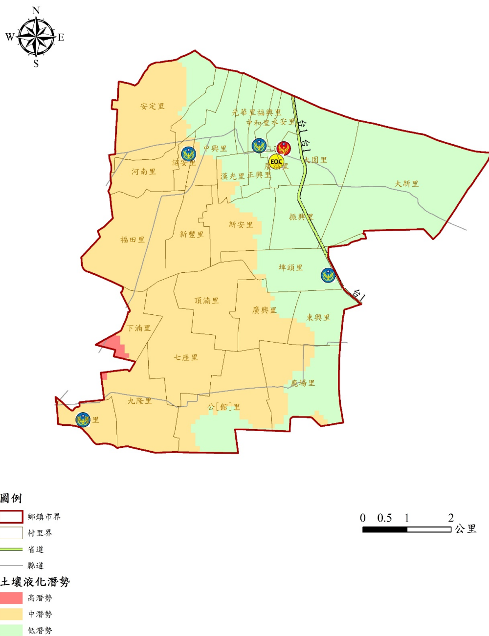
圖 1-4-3 西螺鎮土壤液化潛勢圖
