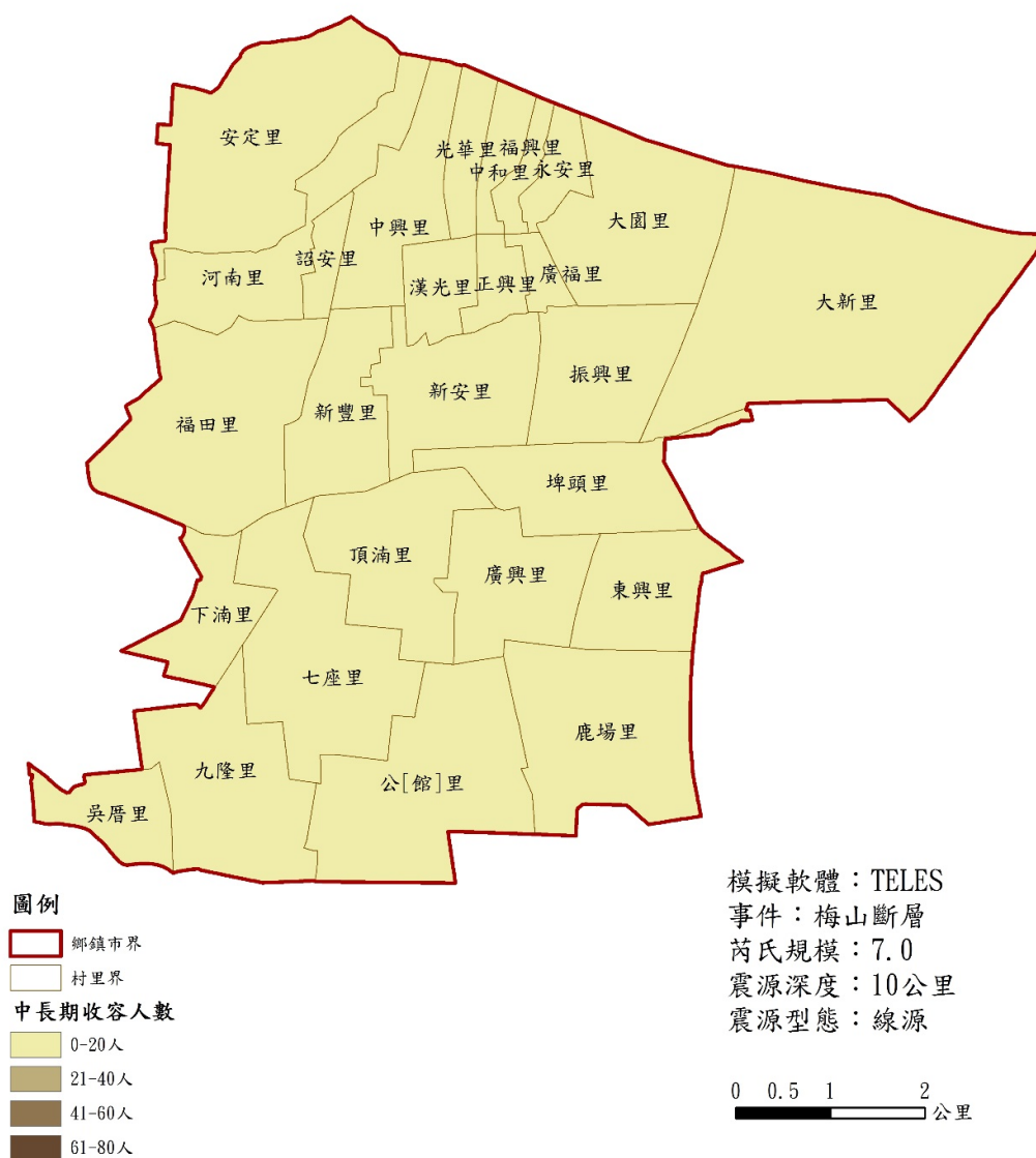
圖 1-4-10 西螺鎮地震災害潛勢圖(需中長期收容人數)
