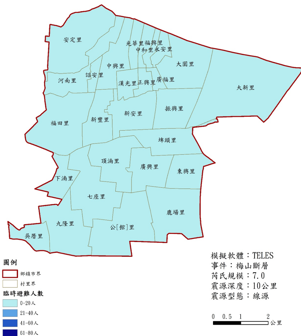
圖 1-4-9 西螺鎮地震災害潛勢圖(需臨時避難人數)
