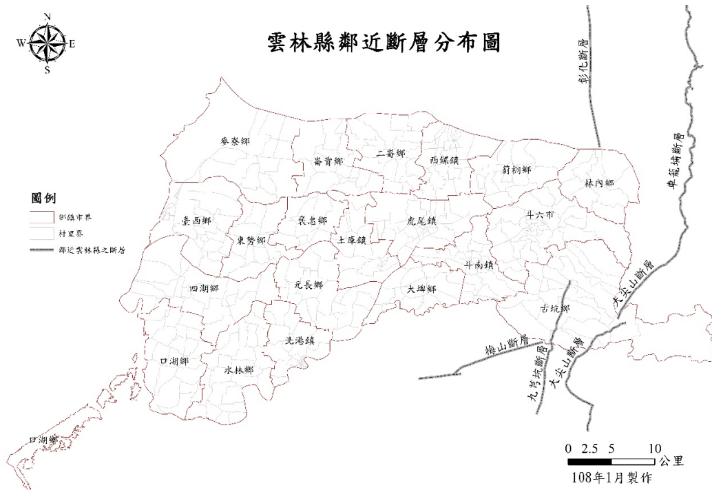
圖 1-4-2 雲林縣鄰近斷層分布圖
