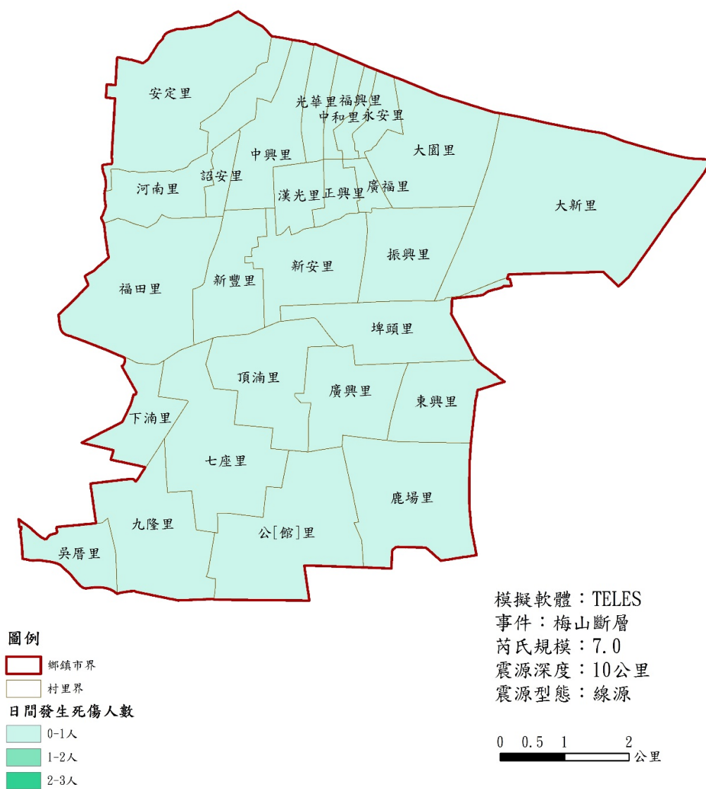
圖 1-4-7 西螺鎮地震災害潛勢圖(傷亡人數-日間)
